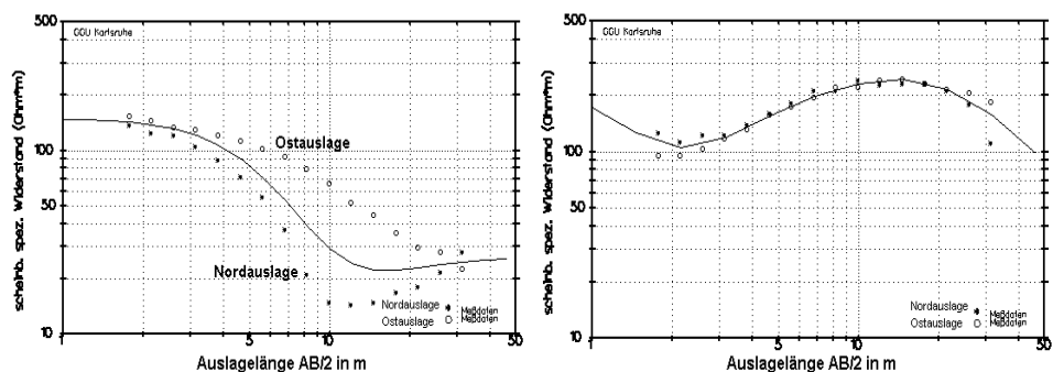
Abb. 3 Daten von 2 Doppel-Widerstandssondierungen. Links: im gestörten Bereich nahe der Deponie mit unterschiedlichen Meßwerten in beide Auslagerichtungen und rechts: im ungestörten Bereich mit nahezu identischen Meßwerten in beide Auslagerichtungen.
