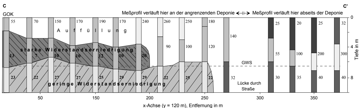
Abb. 4 Tiefenschnitt C - C', ermittelt aus Doppel-Widerstandssondierungen.
