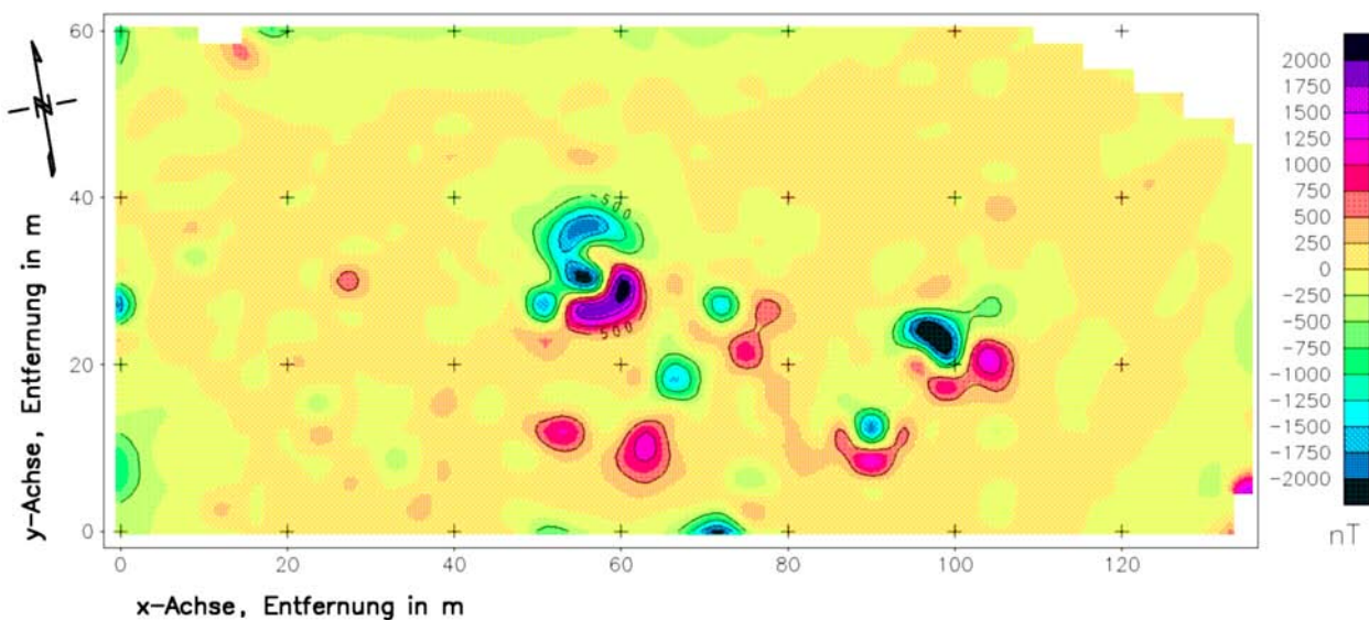
Abb. 1 Anomalienfeld der erdmagnetischen Totalintensität auf der Brachfläche. Die zentral gelegenen Dipolanomalien werden durch die gesuchten Tanks verursacht. Randliche Anomalien kommen durch nahe an der Oberfläche befindliche Eisenobjekte (v.a. Fahrzeuge) zustande.
