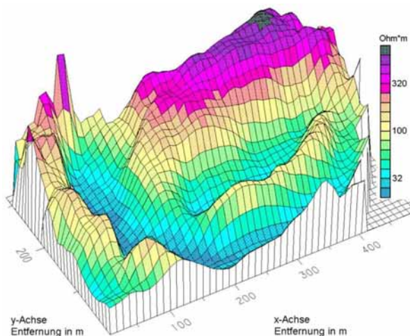
Abb. 3 Dreidimensionale Darstellung des scheinb. spez. Widerstandes, ermittelt durch die Widerstandskartierung. Nach Interpretation durch die Widerstandssondierungen kann dieses Diagramm qualitativ als Tiefendiagramm gelesen werden.
