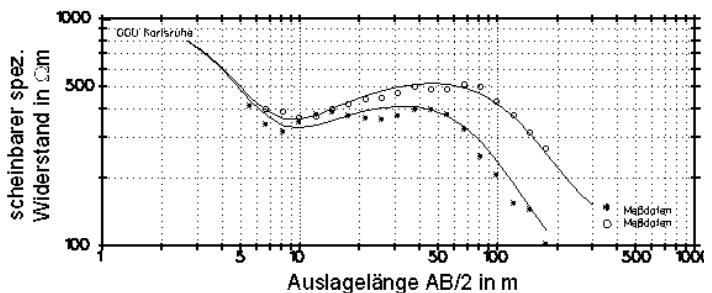
Abb. 3 Daten einer Doppel-Widerstandssondierung in zwei Auslagerichtungen Kreise und Sternchen: Meßdaten getrennter Richtungen Linien: synthetische Daten des jeweiligen Tiefenmodells
