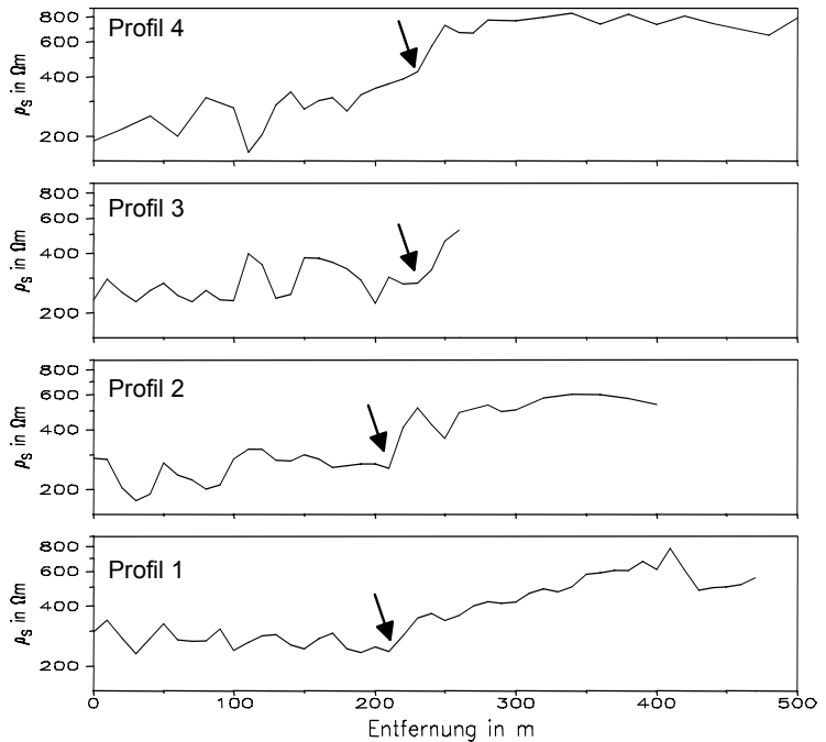
Abb. 1 Vier parallele Widerstandsprofile
