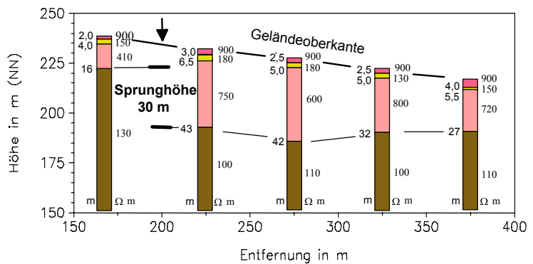
Abb. 2 Tiefendiagramme von 5 Widerstandssondierungen
