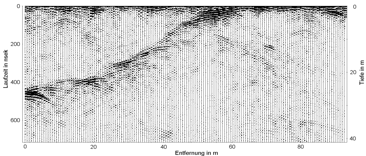
Abb. 3 100 MHz-Radargramm einer Meßlinie entlang der Stollensohle mit Strahlrichtung vertikal nach unten (Meßposition S in Abb. 2). Zur Berechnung der Tiefenachse wurde die Dielektrizität des Dolomits mittels spezieller Meßgeometrie (CMP) sowie aus Beugungserscheinungen (Diffraktionen) zu \epsilon = 6,6 bestimmt. Aus der Reflexionslaufzeit und der Dielektrizität läßt sich die Tiefen der Reflektoren berechnen.
