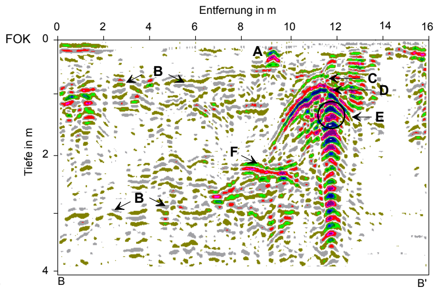
Abb. 4 Radargramm/Schnitt B - B' Interpretationen: A Leitung B Bodenschichten C Gewölbeoberkante D Unterkante des Mauerwerks E metallisches Objekt im Hohlraum F Schichtgrenze
