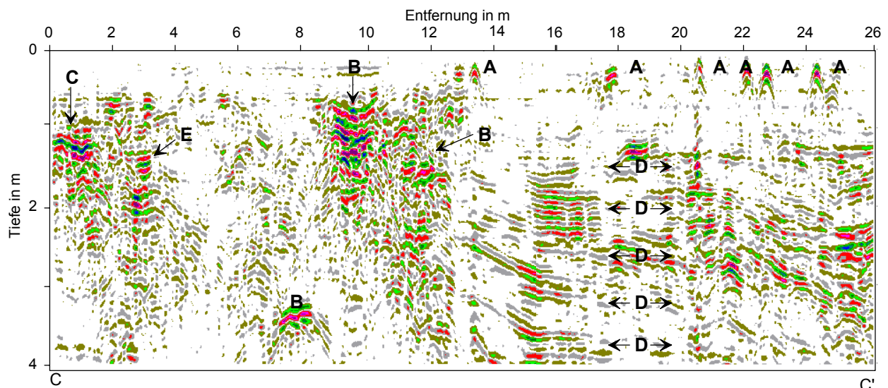
Abb. 5 Radargramm/Schnitt C - C' Interpretationen: A Leitungen B Gräber C Gewölbe (siehe Schnitt A - A') D Bodenschichten E Mauer
