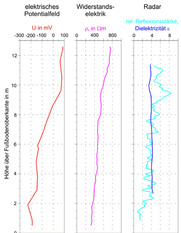
Abb. 3 Meßergebnisse an einem Pfeiler
