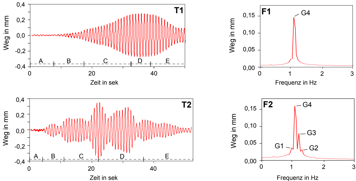
Abb. 2 Schwingwege und -frequenzen
