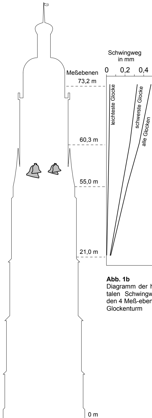
Abb. 1a Glockenturm mit 4 Glocken und 4 Meßebenen der Schwingungsuntersuchungen
